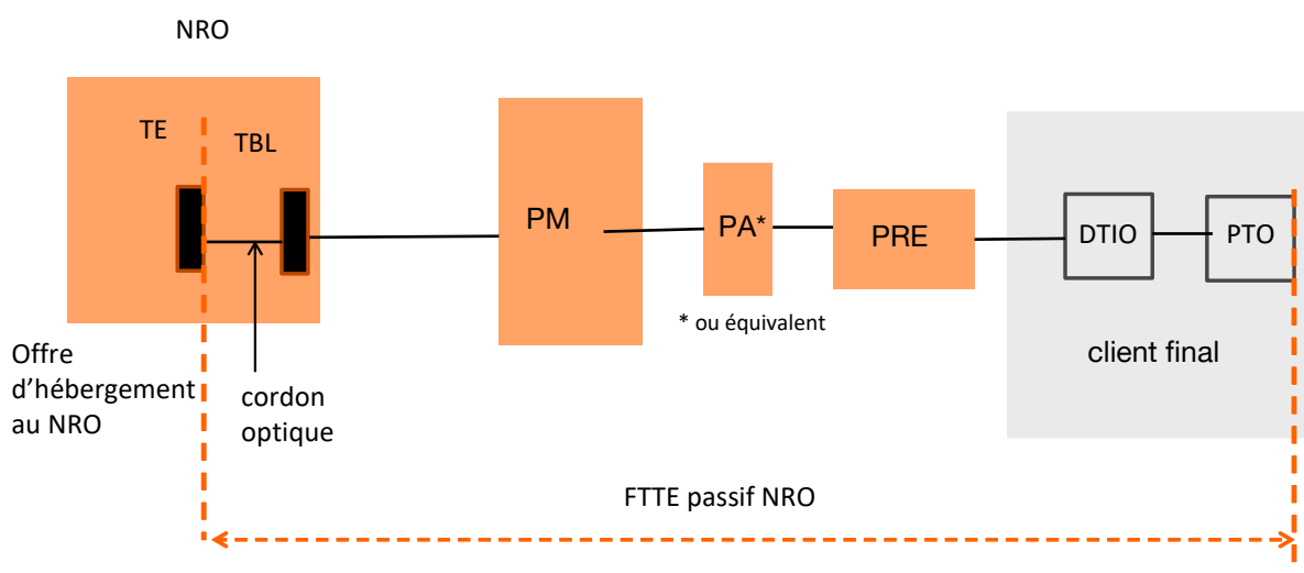
Figure 1 : Synoptique de l'Accès FTTE passif NRO
